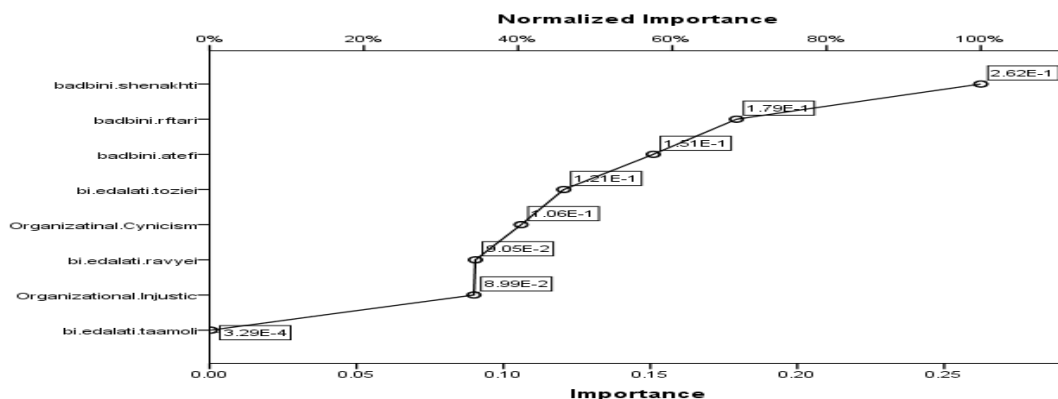
شکل ۳. میزان اهمیت متغیرها در پیش‌بینی طفره‌روی مجازی به روش شبکه عصبی مصنوعی
