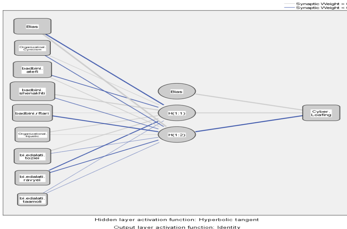
شکل ۲. وزن‌های سیناپسی و لایه‌های شبکه عصبی
